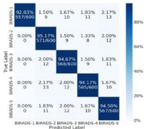
Hình 5.5. Ma trận nhầm lẫn
